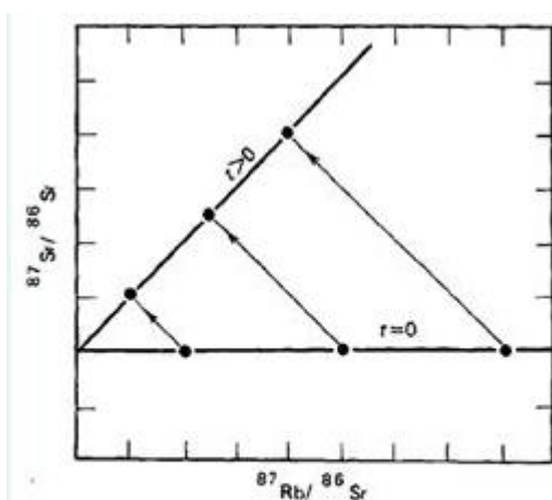
Рис. 8.1. Rb-Sr изохронная диаграмма, показывающая изотопную эволюцию пород во времени после их кристаллизации из гомогенной магмы.
